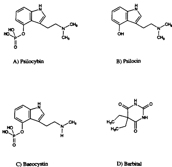
Fig. 1. Structures of (A) psilocybin, (B) psilocin, (C) baeocystin and (D) barbitol.
